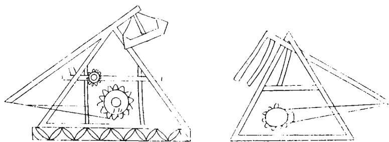
106. Орудіе для метанія Греческаго огня.
